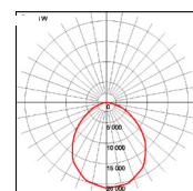
300W-5000K-50°x90°
